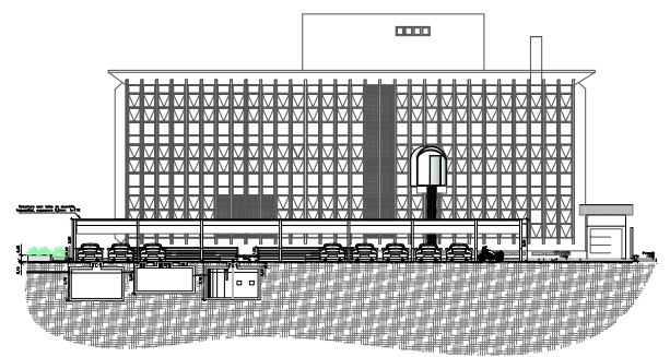
CORTES B.B.
