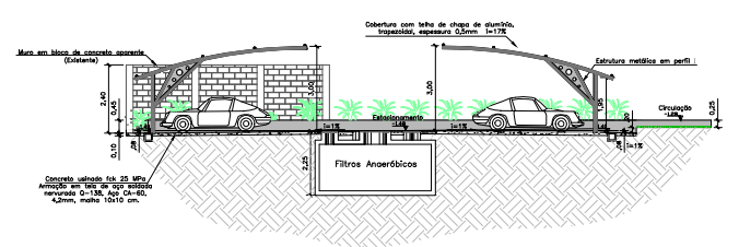
CORTES A.A.
