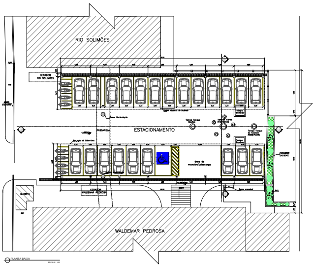
PLANTA B.004
